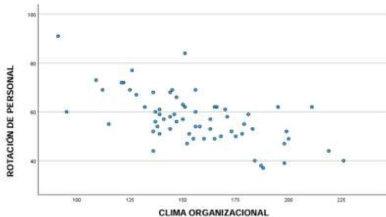
Figura 4 Correlación entre clima organizacional y rotación de personal
